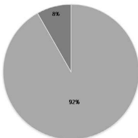
OY 2013 Enplanements 1/
